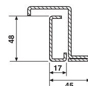
Telaio Ridotto con Microfalso
