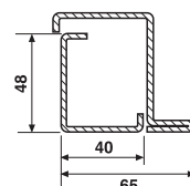
Telaio Ridotto con Falsotelaio Ridotto
