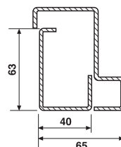
Telaio Normale con Falsotelaio Normale
